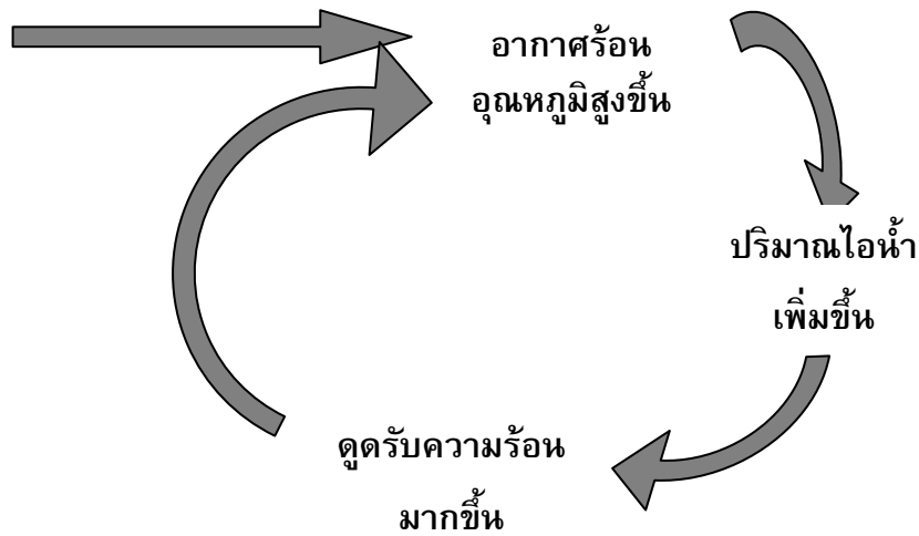
รูปที่ 2.1 ไอน้ำทำหน้าที่ดูดซับความร้อน เมื่อมีปริมาณไอน้ำเพิ่มขึ้น การดูดซับความร้อนในบรรยากาศก็เพิ่มมากขึ้นด้วย ทำให้บรรยากาศของโลกมีอุณหภูมิสูงขึ้น
